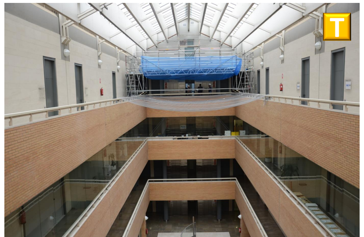
Edificio Realia (Sevilla) estructura móvil librando hueco de patio y adaptada a la pendiente a dos aguas de la cubierta.
