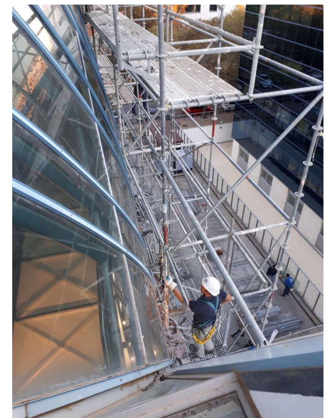
Estructura multidireccional para trabajos sobre bóveda y lucernario tanto por el interior como por el exterior del edificio.
