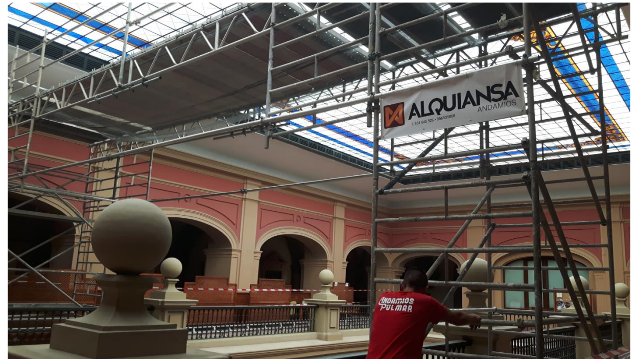
Rectorado de Sevilla (Real Fábrica de Tabacos) estructura móvil sobre railes librando hueco de patio.
